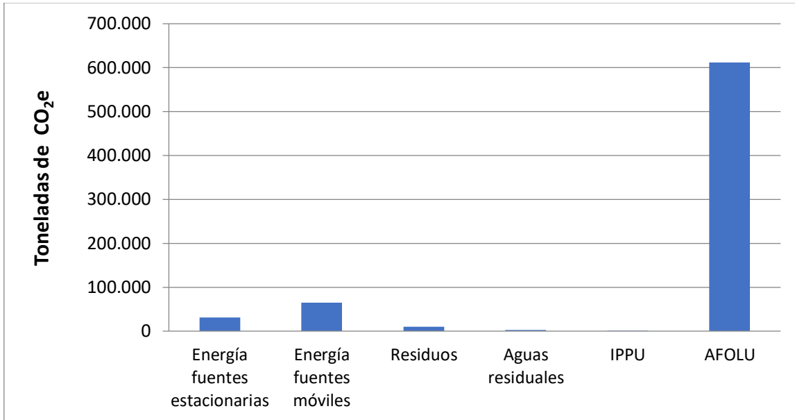
Figura 24. Principales emisiones de GEI en 2016
