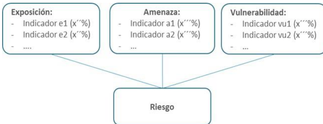
Figura 20. Análisis de riesgos climáticos en función de la exposición, vulnerabilidad y amenaza
