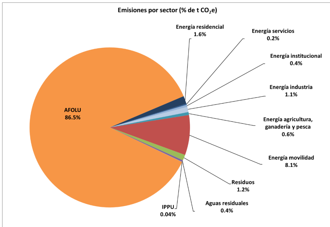
Figura 4. Emisiones totales de GEI del inventario del municipio de Cocula de 2016 desagregado por sector
