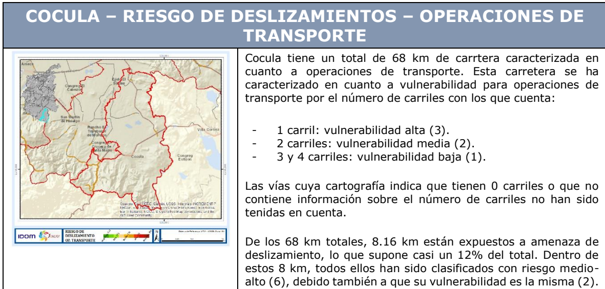
Figura 19. Riesgo de deslizamiento en operaciones de transporte
