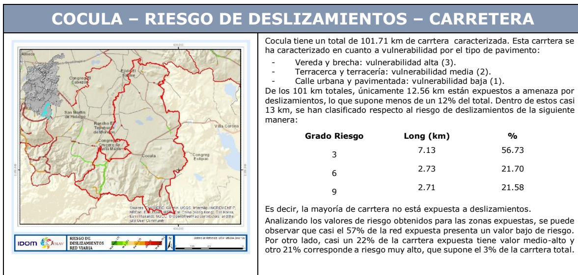
Figura 18. Riesgo de deslizamientos en carretera
