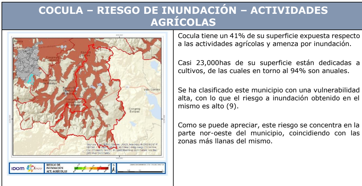
Figura 10. Riesgo de inundación en viviendas
