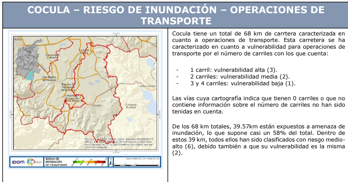
Figura 13. Riesgo de inundación en las operaciones de transporte
