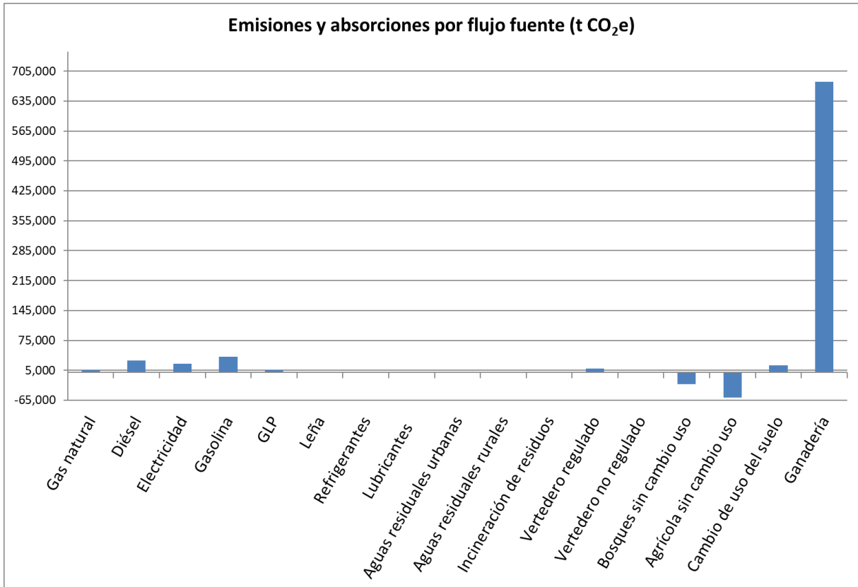
Figura 5. Balance de emisiones de GEI del inventario del municipio de Cocula de 2016 desagregadas por flujo fuente (t CO 2 e)
