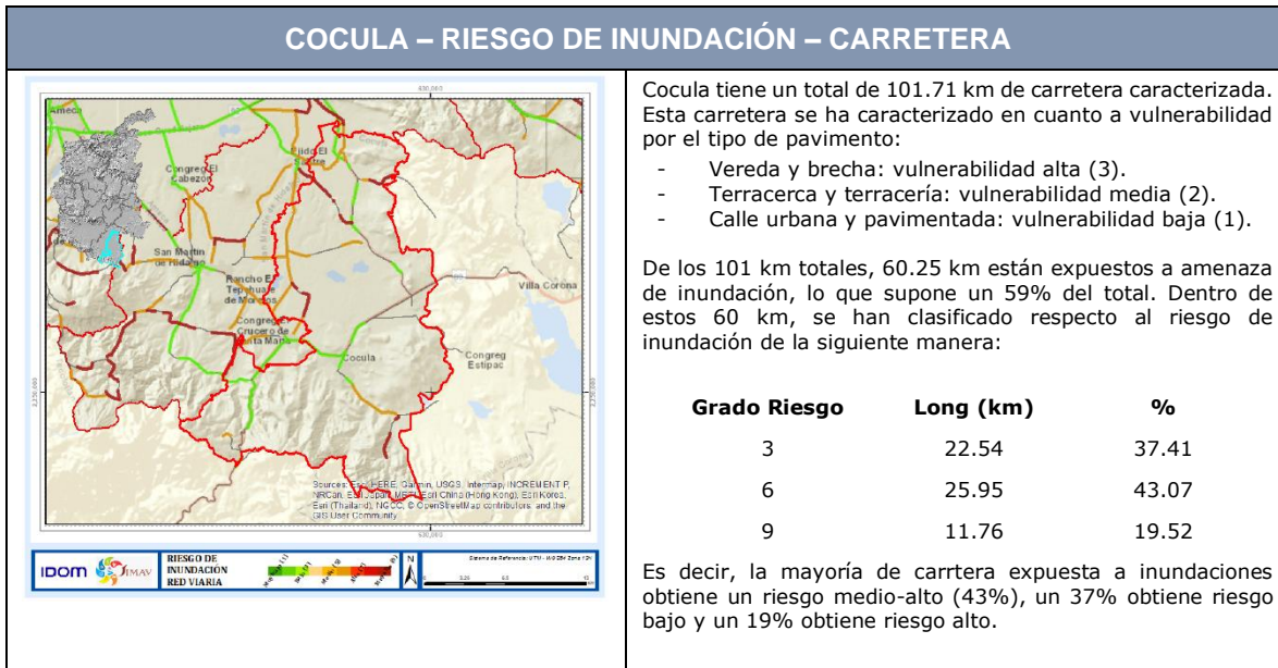
Figura 12. Riesgo de inundación en carreteras
