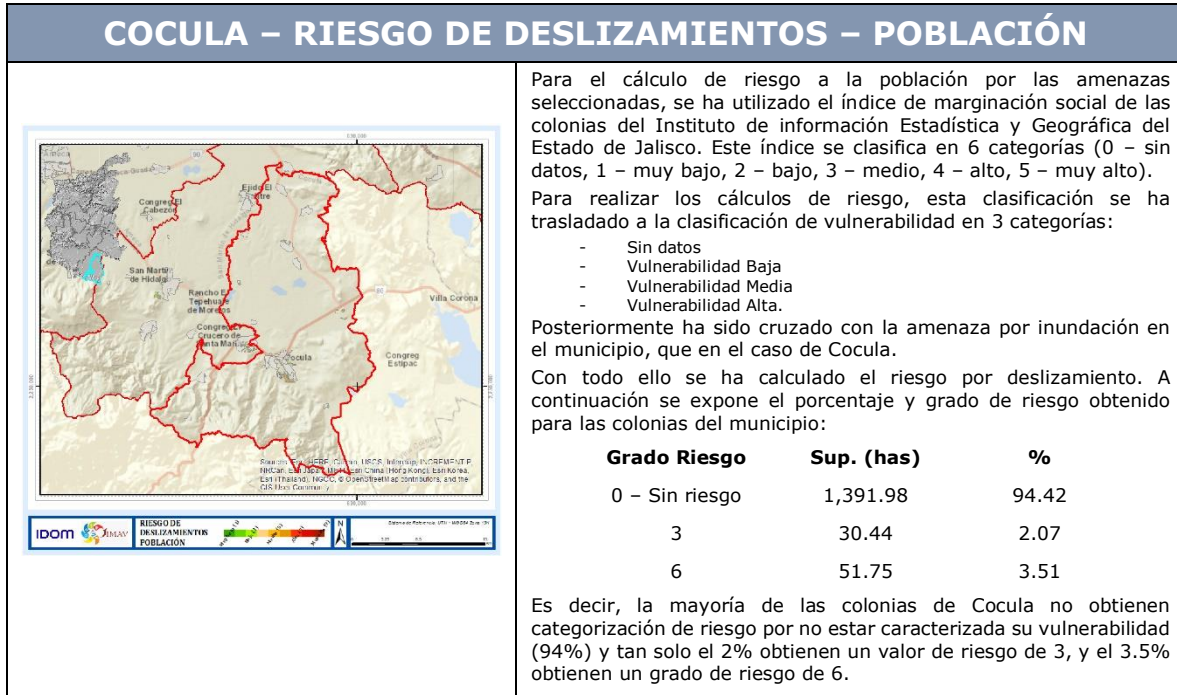
Figura 17. Riesgo de deslizamientos en la población
