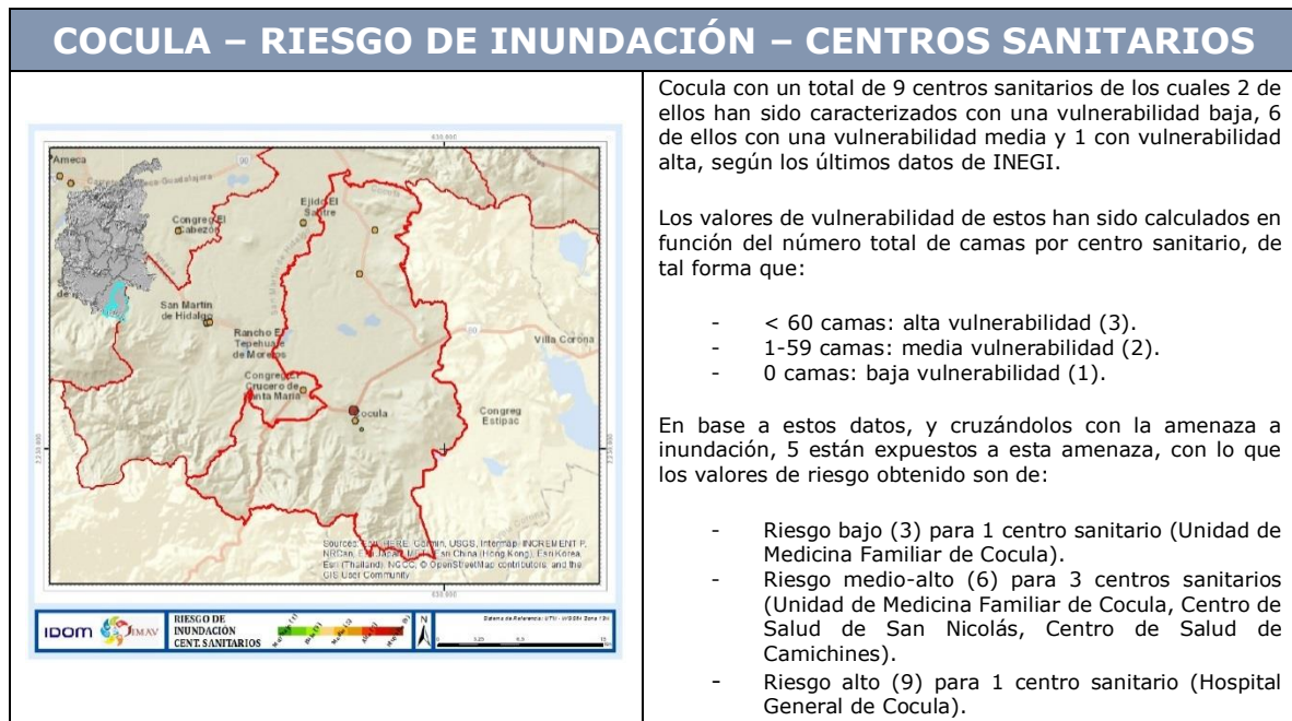
Figura 14. Riesgo de inundación en centros sanitarios
