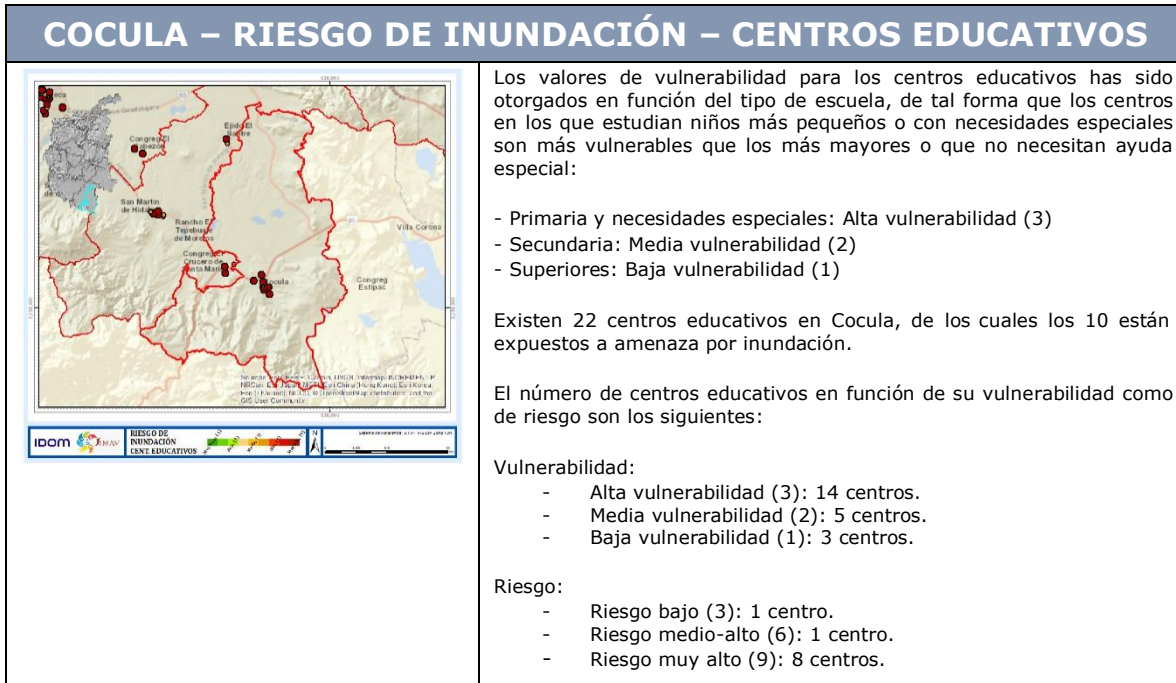
Figura 15. Riesgo de inundación en los centros educativos
