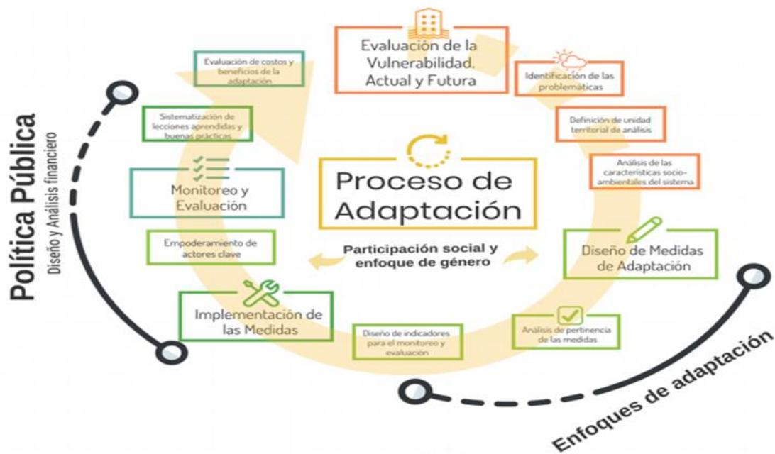
Figura 27. Proceso de adaptación al cambio climático
